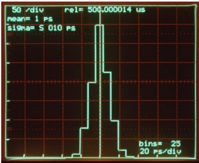
Histogram display
